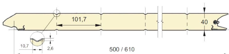
Nové rozměry rozestupu jednotlivých drážek designu Lamela
